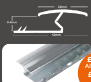
Zig Zag® 9mm - M34
